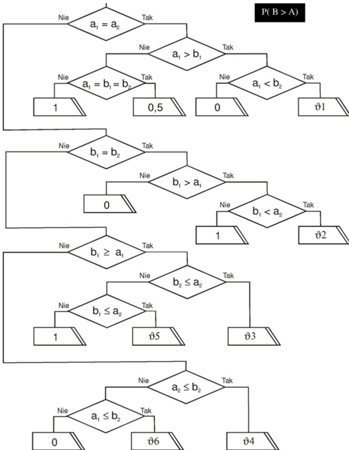
Rys. 4.2. Schemat blokowy operatora porównywania przedziałów [ a_1 , a_2 ] i [ b_1 , b_2 ]
